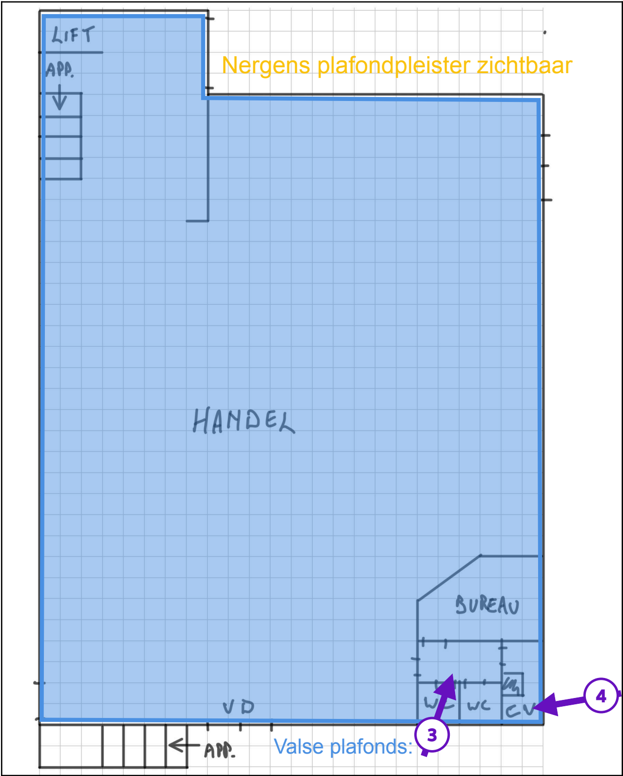
Legende van plan 1.5: Handelsruimte gelijkvloers
